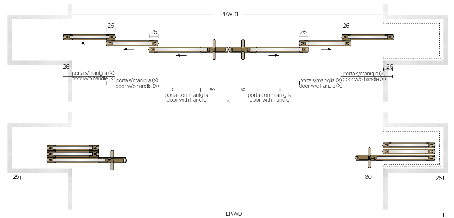
DOUBLE OPENING WITH 2 RECESSED COMPARTMENTS APERTURA DOPPIA CON 2 VANI AD INCASSO
