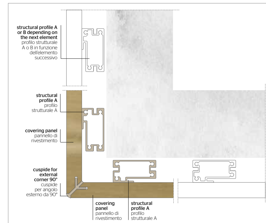
90° external corner Composition with two linear panels Angolo esterno 90° Composizione realizzata con due pannelli lineari
