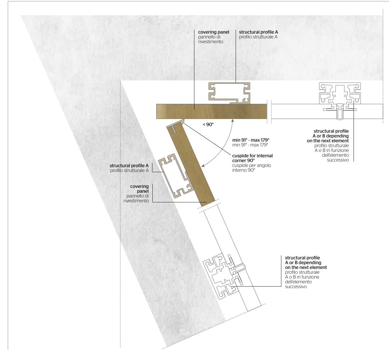
< 90° internal corner Composition created with two linear panels Angolo interno < 90° Composizione realizzata con due pannelli lineari
