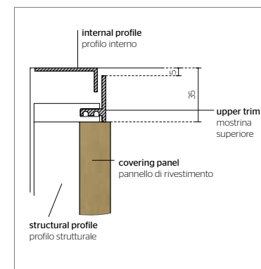
detail C dettaglio C
