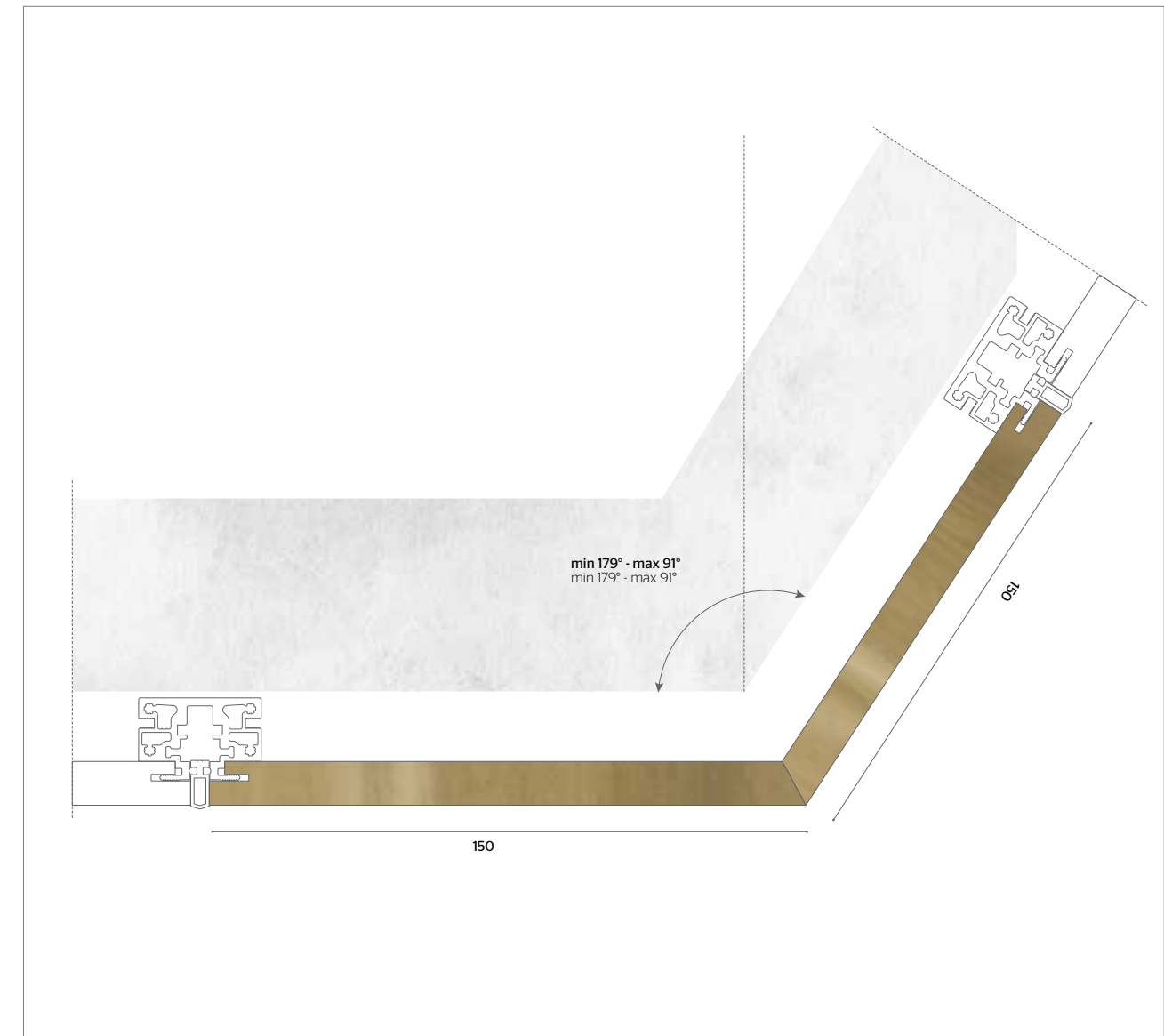
> 90° external corner Composition with two linear panels Angolo esterno > 90° Composizione realizzata con due pannelli lineari
