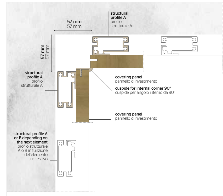
90° internal corner Composition with two linear panels Angolo interno 90° Composizione realizzata con due pannelli lineari
