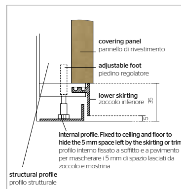
detail D dettaglio D
