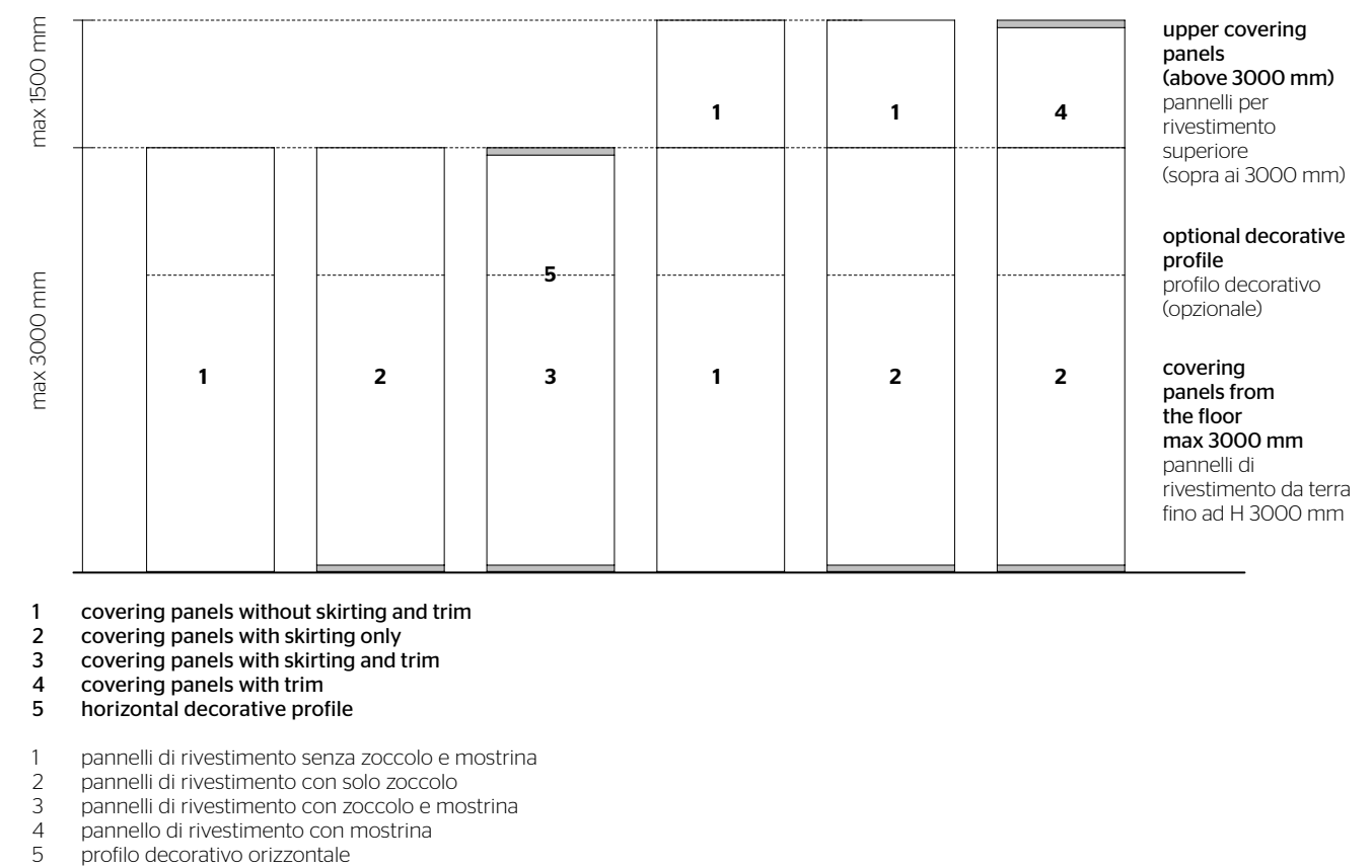
Covering panels front view with horizontal decorative profile Vista frontale pannelli di rivestimento con profilo decorativo orizzontale
