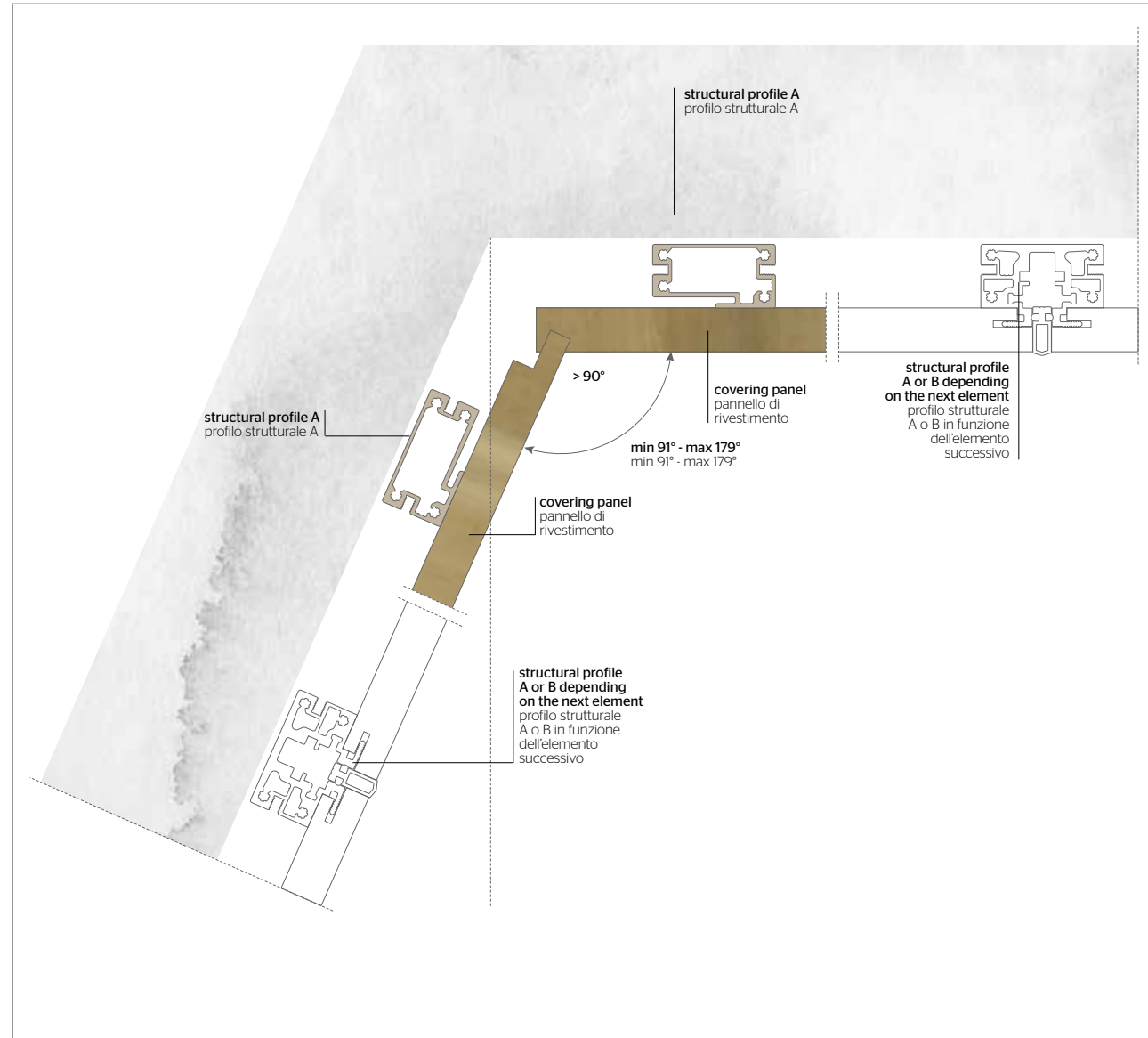
> 90° internal corner Composition with two linear panels Angolo interno > 90° Composizione realizzata con due pannelli lineari
