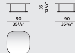
SQUARE COFFEE TABLE TAVOLINO QUADRATO
