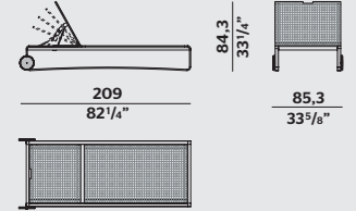
SUNBED BATYLINE VERSION LETTINO VERSIONE BATYLINE
