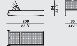
SUNBED WOVEN ROPE VERSION LETTINO VERSIONE INTRECCIO
