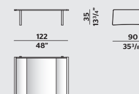
LAVA STONE TOP COFFEE TABLE TAVOLINO PIANO PIETRA LAVICA
