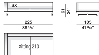
end element TE225A dx - sx
