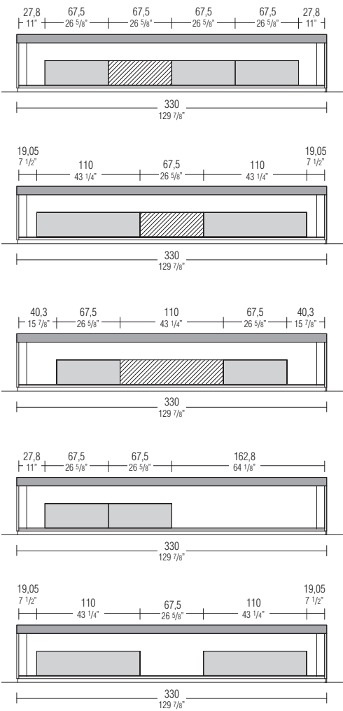
W 330 - 129 7/8"
