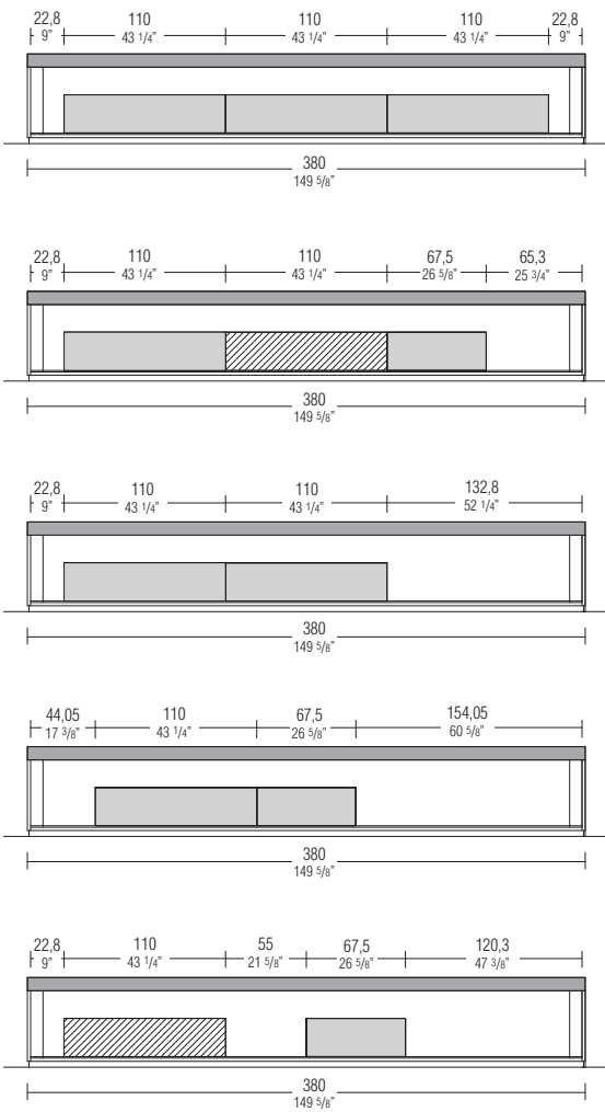
W 380 - 149 5/8"
